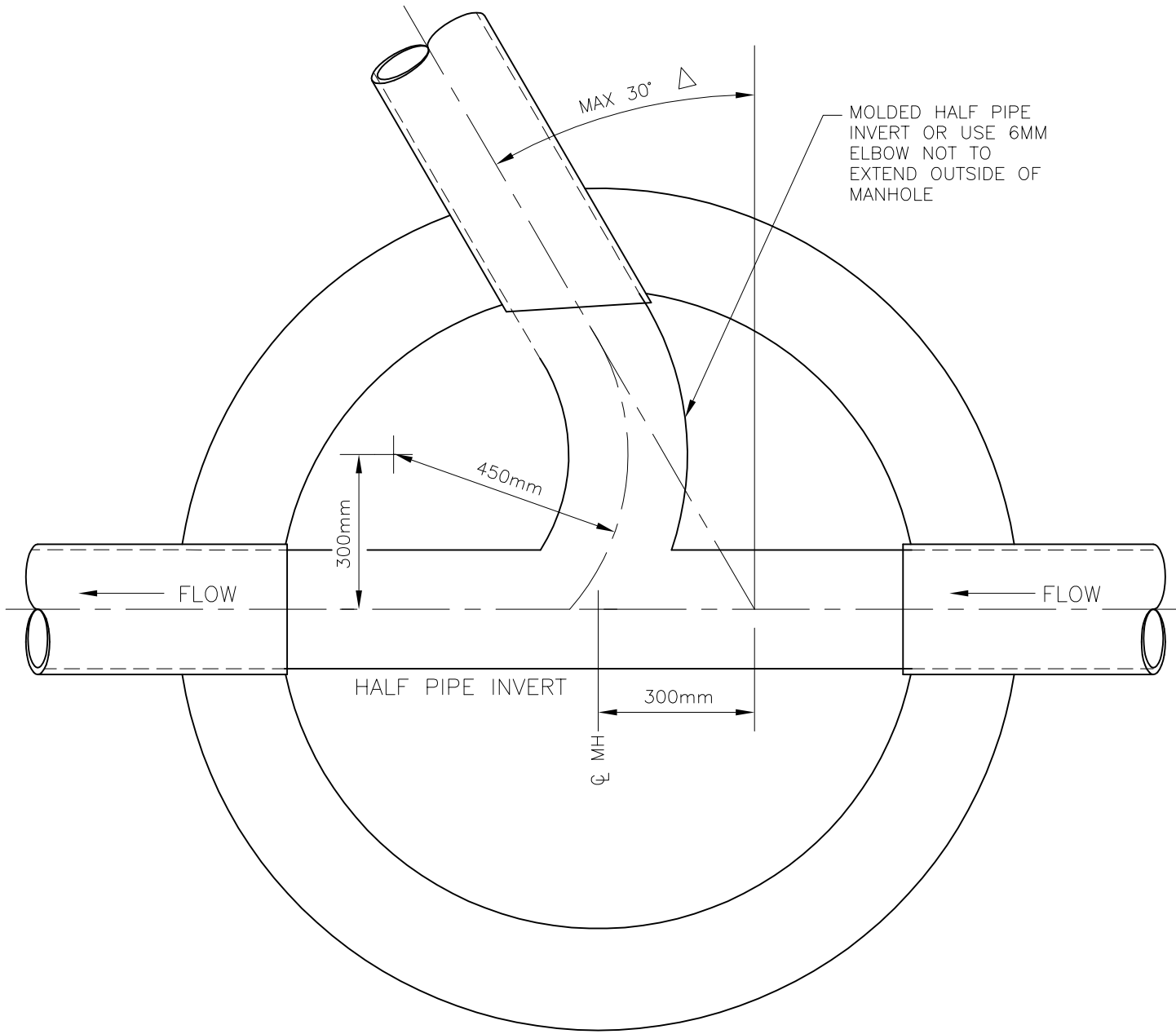
STANDARD 1220 A MANHOLE
