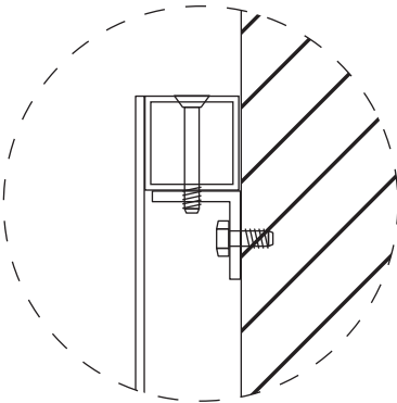
Detail C Scale: NTS
